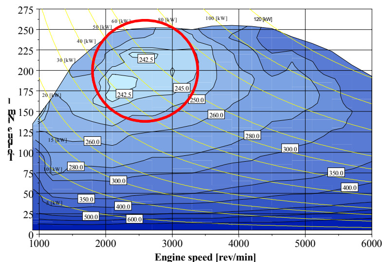
Figure 3.1 : schéma du moteur sur une voiture à essence récente de catégorie moyenne
